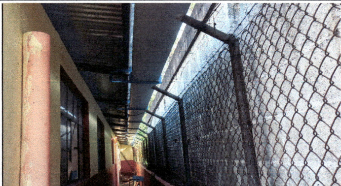
Foto 1: En módulo 1, se observa canal de de lámina lisa, instalada, con sus respectivos pescantes.
